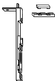
Ref. 0300-D1 Ref. 0300-D3 Pasador Metálico y Cerrojillo
